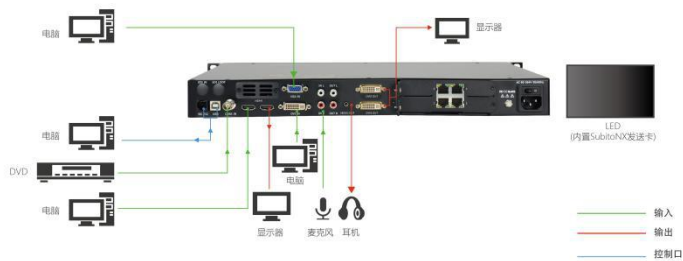
图为 X1Gpro 的系统连接简图
