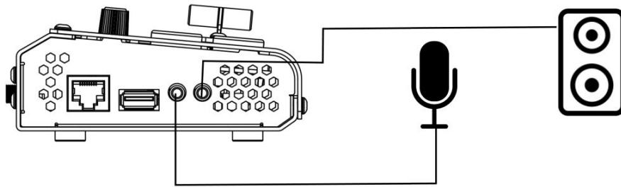
将麦克风和音箱连接至 mini 的 AUDIO IN/OUT
