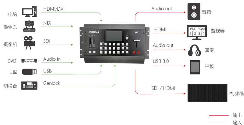
M1 的系统连接简图
