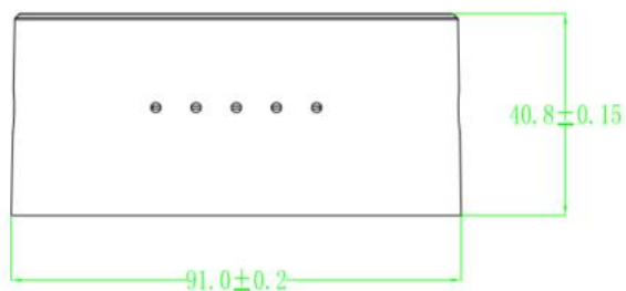
右视图
