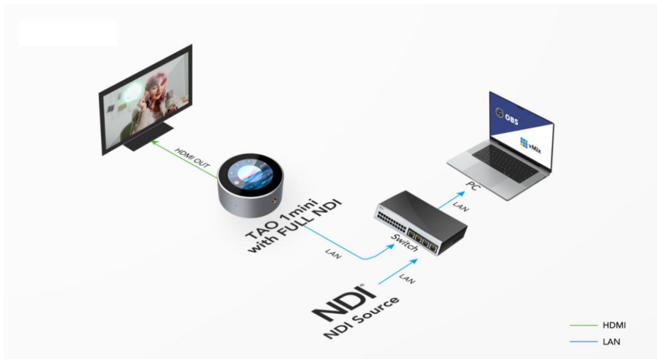
NDI 解码应用方案图
