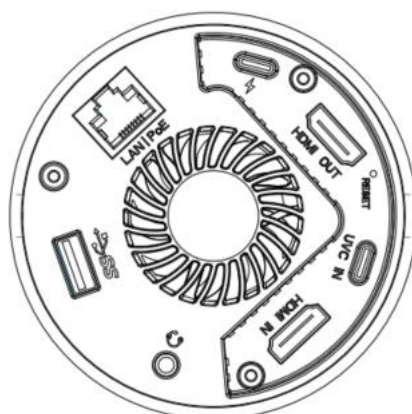
后视图
