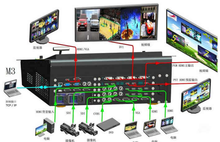
图为 M3 视频处理器的系统连接简图
