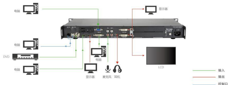
图为X1Gpro的系统连接简图
