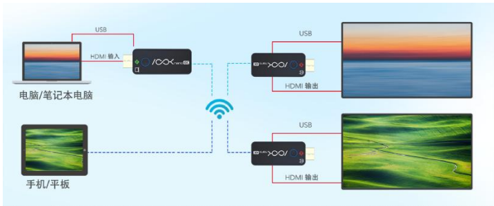
ASK nano 4K（1 发 2 收）系统连接简图 2
